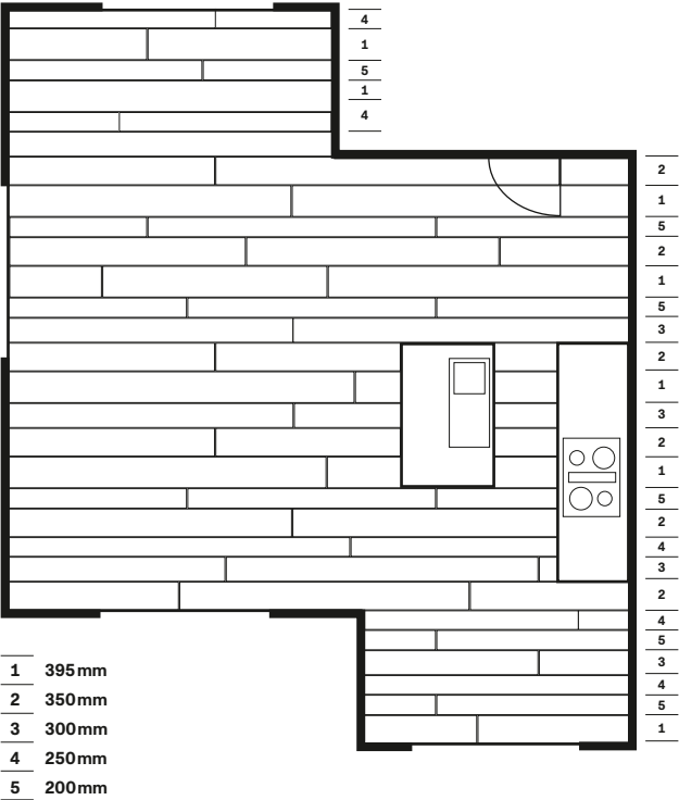
Exemple de plan sur une échelle de 1:100
