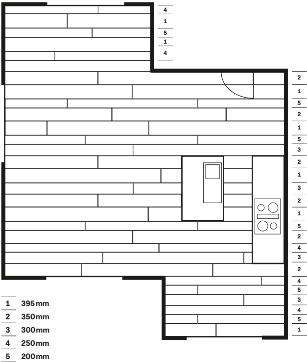
Beispiel Grundriss-Plan im Massstab 1:100
